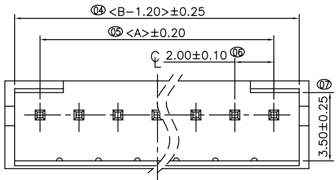
3P以上视图
