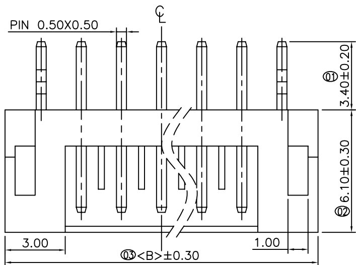
3P以上视图
