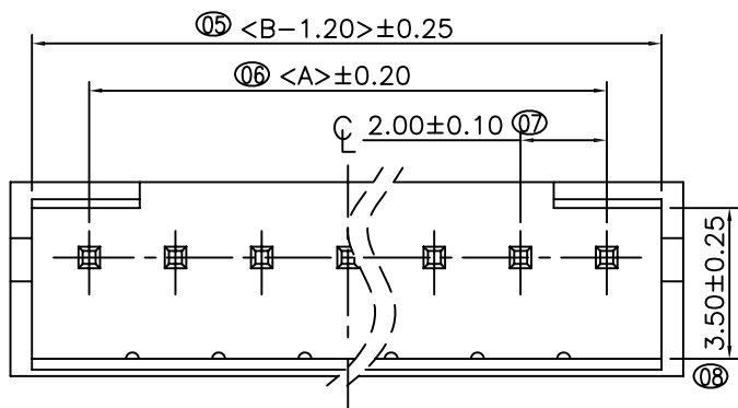
3P以上视图
