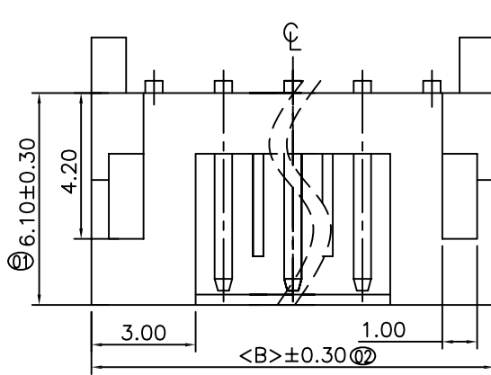
(3 Pin 以上视图)
