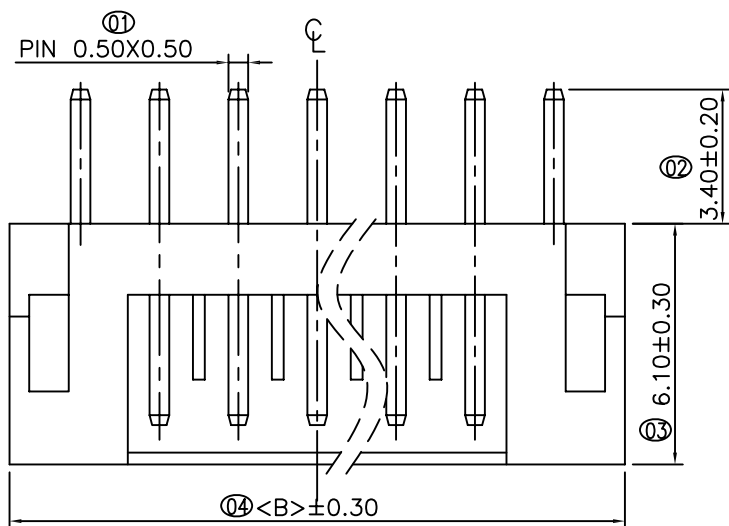
3P以上视图
