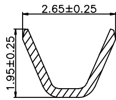
SEC:A-A
