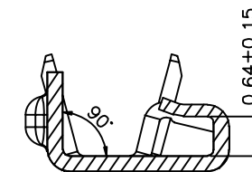
SEC:D-D
