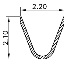
A-A SECTION
