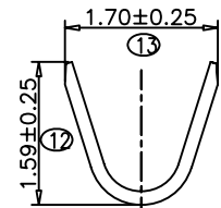
SECTION:A-A SCALE 1:1
