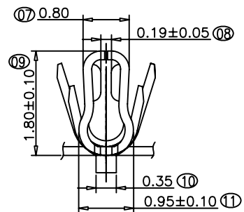
SECTION:B-B SCALE 1:1
