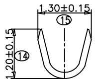
SECTION:B-B SCALE 1:1
